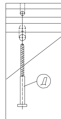
Крепление винта саморезного (компл.№19)
